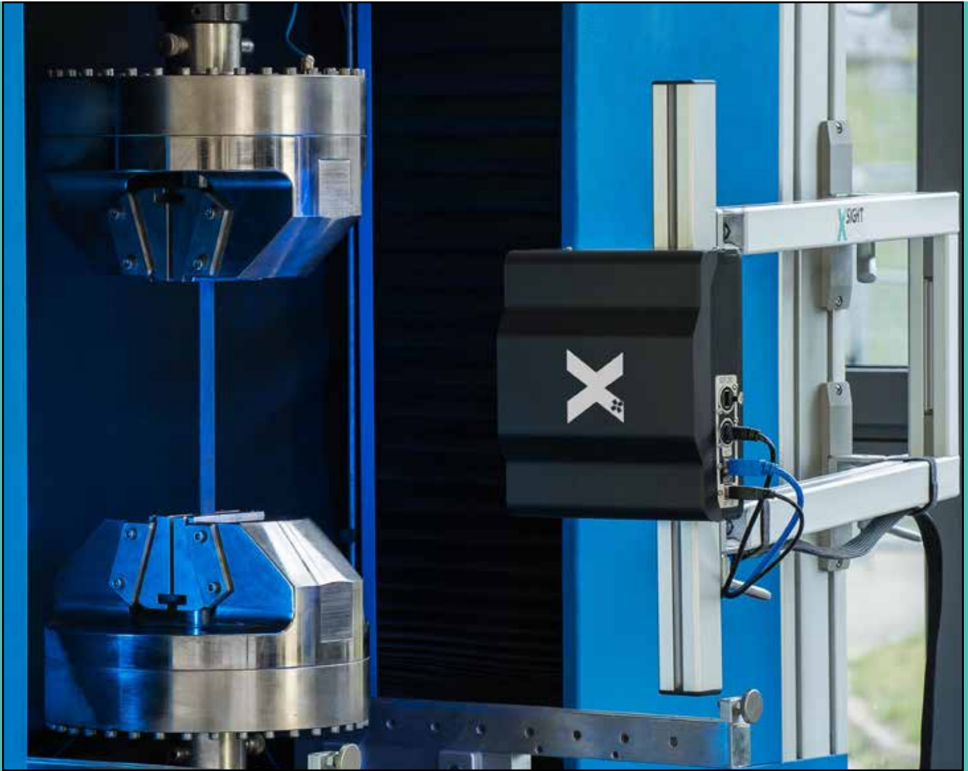
TENSILE TESTING
